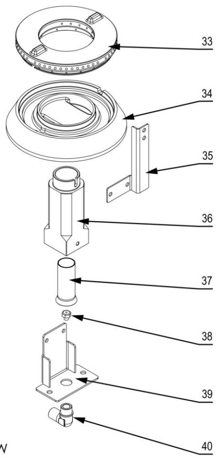
Palnik 5kW
