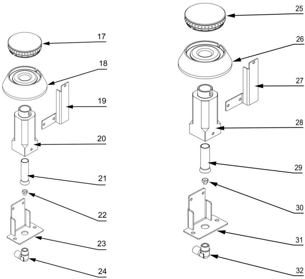
Palnik 5kW
